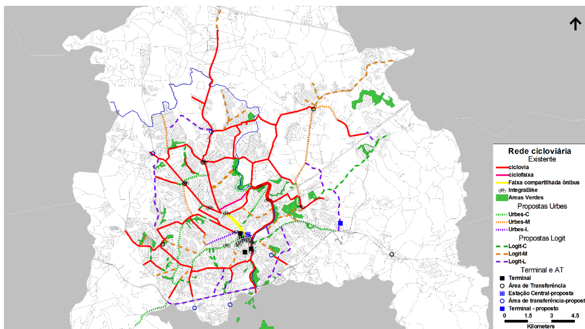
Figura 60: Rede Ciclovária Proposta (Fonte: Análise Logit)
