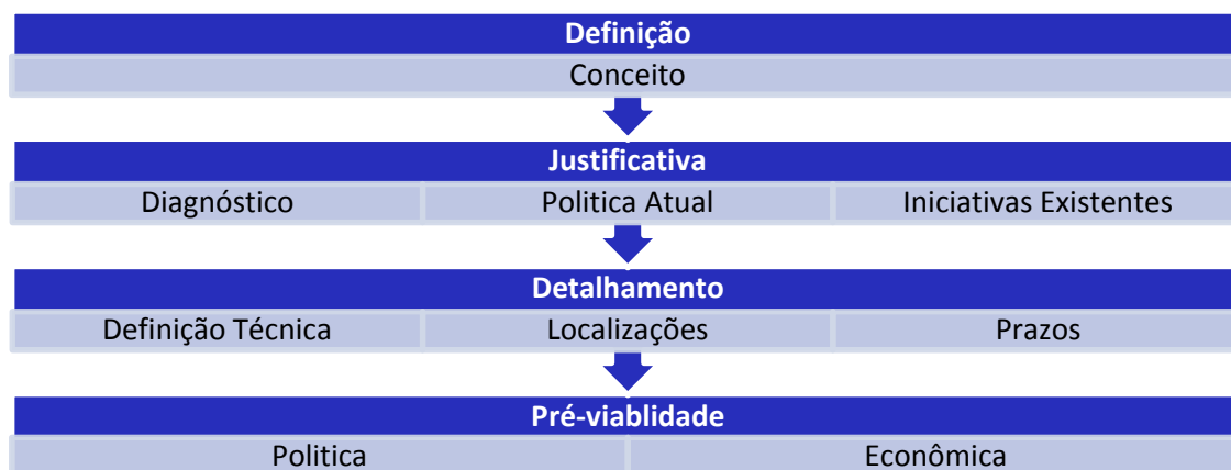
Figura 17: Metodologia Aplicada
