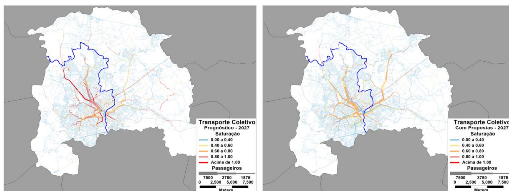
Figura 77: Carregamento - Comparação Prognóstico e Proposta (2027) (Fonte: Análise Logit)
