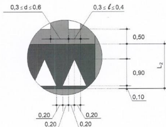
DETALHE A
