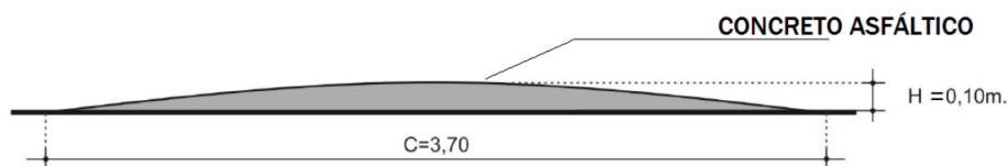
CORTE A-A
