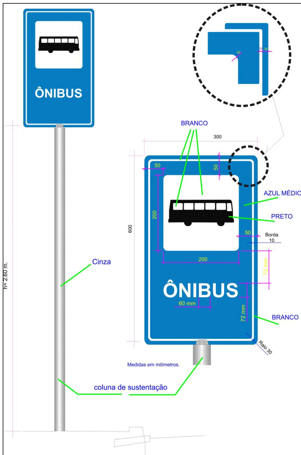
Figura 1. Placa Indicativa de Parada de Ônibus
