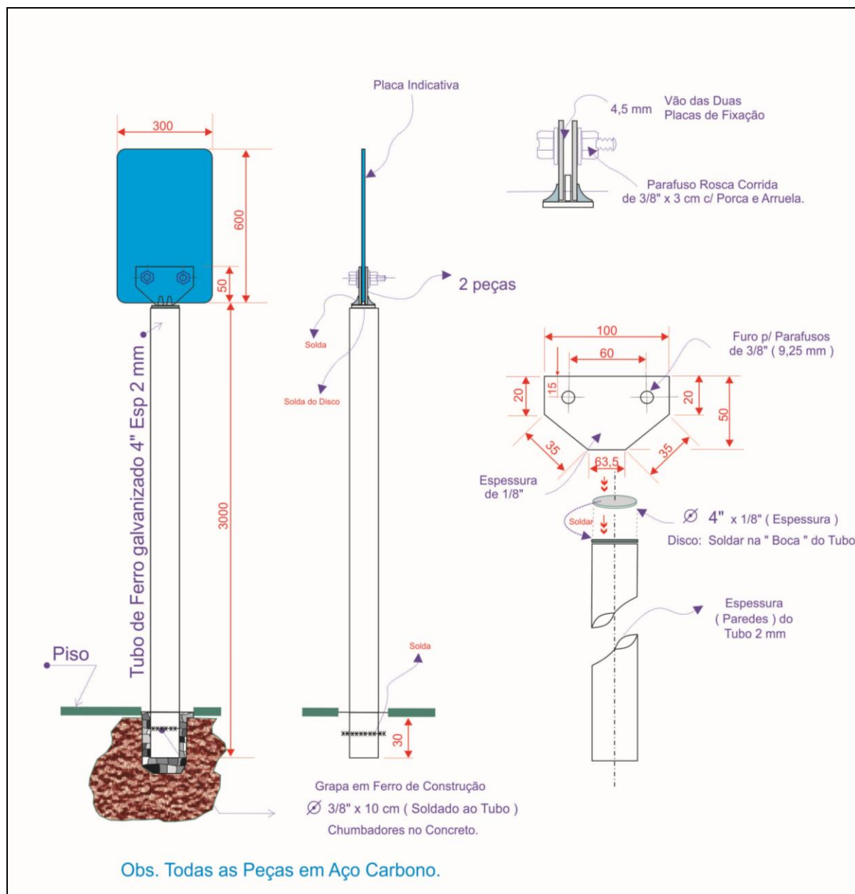
Figura 2. Poste de Sustentação
