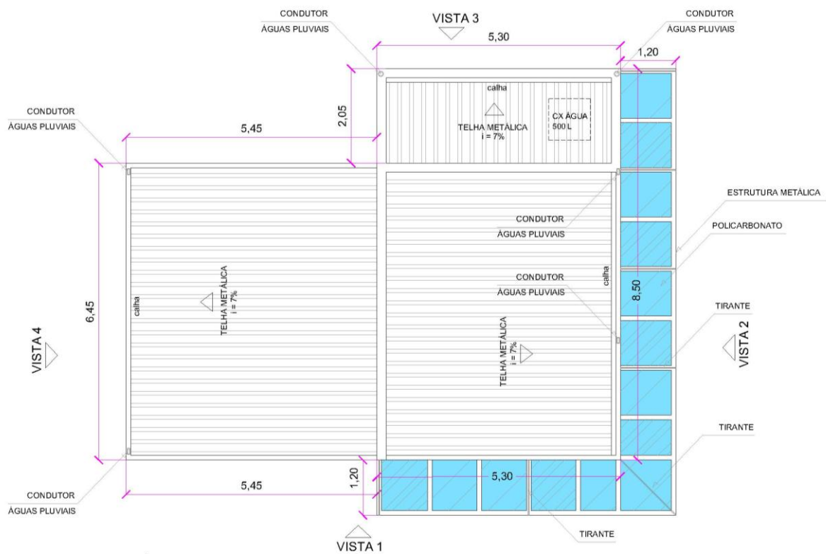
MÓDULO TIPO 02 PLANTA COBERTURA
