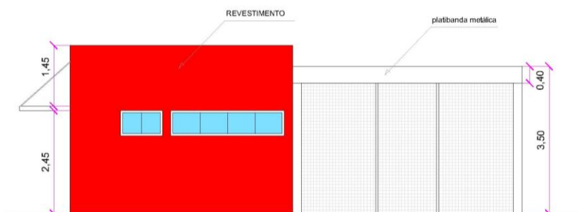
VISTA 3 MÓDULO TIPO 02
