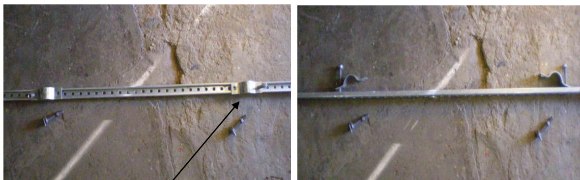
Abraçadeiras de 3” ou 4”
